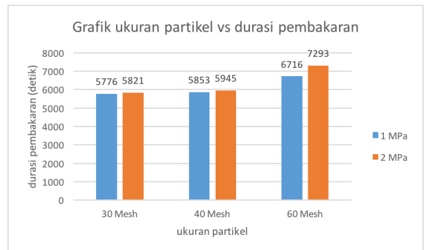
Gambar 11 Pengaruh ukuran partikel terhadap durasi pembakaran
