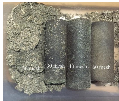
Gambar 7 Briket dengan tekanan press 20 bar (2MPa)
