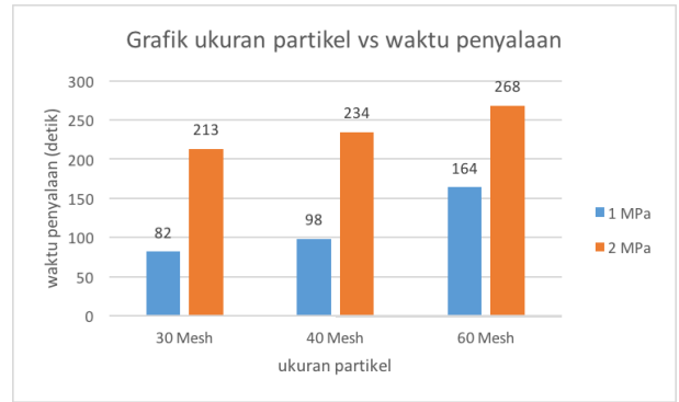
Gambar 10 Pengaruh ukuran partikel terhadap waktu penyalan
