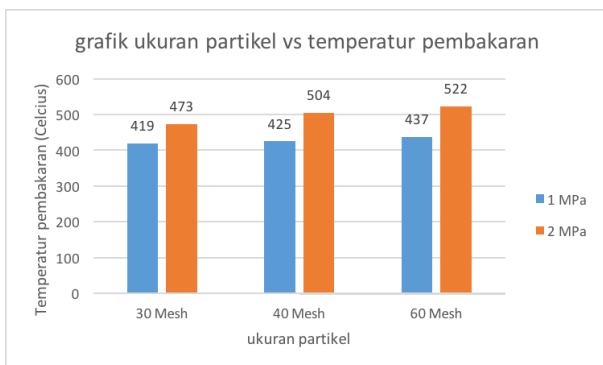
Gambar 9 Pengaruh ukuran partikel terhadap temperatur pembakaran
