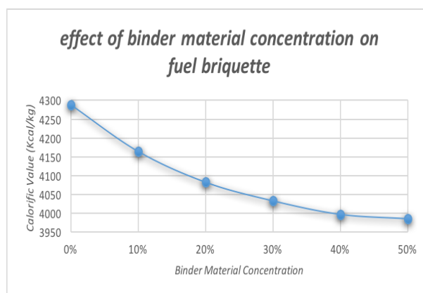
Gambar 8 Grafik nilai kalor terhadap zat perekat
