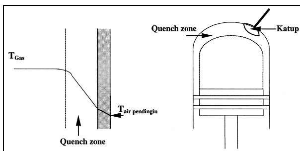
Gambar 1. Quench Zone antara Torak dan Silinder Motor Bakar
