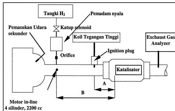
Gambar 7. Skema Pengujian Sistim
