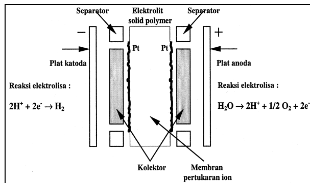
Gambar 3. Konfigurasi dari Sistim Elektrolisa Air dengan Elektrolit Solid Polymer
