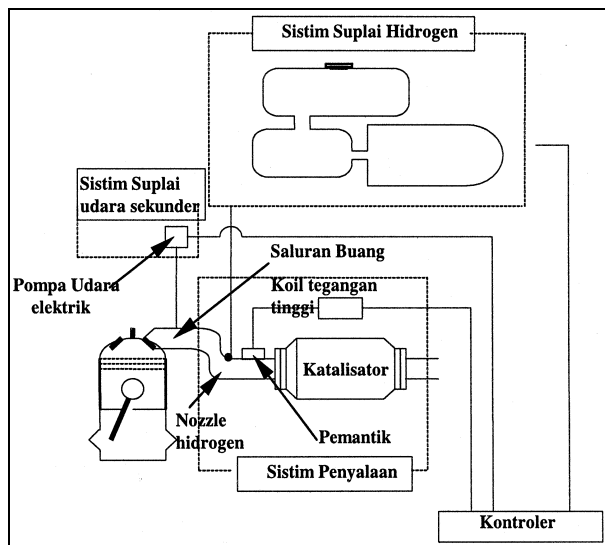
Gambar 6. Spesifikasi Dan Konfigurasi Sistim
