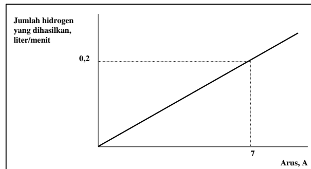
Gambar 5. Kurva Arus yang Digunakan vs Jumlah Hidrogen yang Dihasilkan
