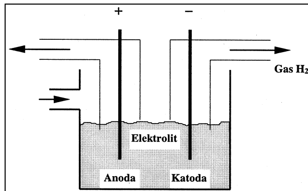
Gambar 2. Skema Prinsip Produksi Hidrogen Dengan Elektrolisa
