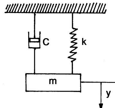
Gambar 1. Sistem Pegas-Peredam Kejut-Massa (diadopsi dari referensi 4 dan 5).
