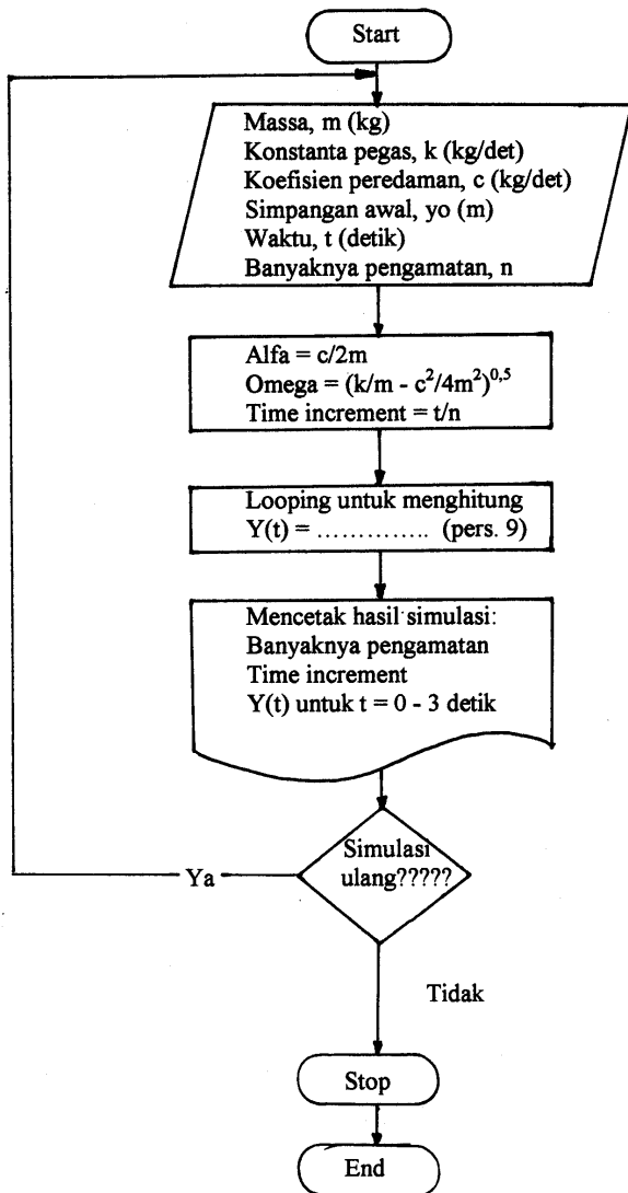
Lampiran 1. Bagan alir program simulasi sistem pegas-peredam kejut-massa
