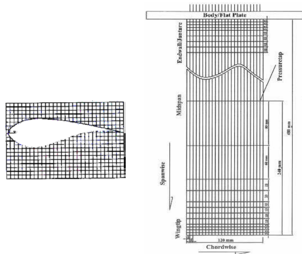
Gambar 6. Posisi Sensor Tekanan pada Airfoil dan Plat Datar
