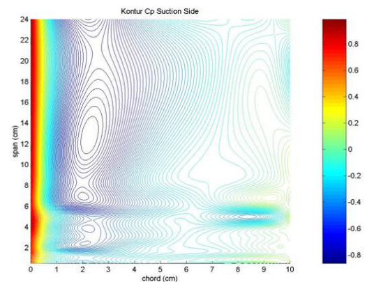
Gambar 29. Kontur Cp Eksperimental Sisi Atas
