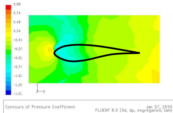
Gambar 19. Kontur C_p di Dinding
