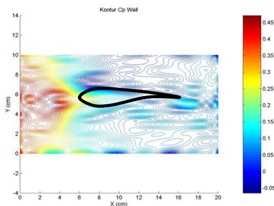
Gambar 31. Kontur Cp Eksperimental di Dinding
