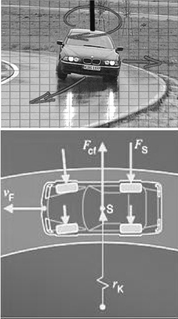
Gambar 2 Efek Gaya Lateral pada Kendaraan
