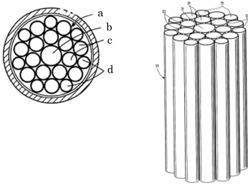
Gambar 1. Tube Bundle dengan 22 Tabung
