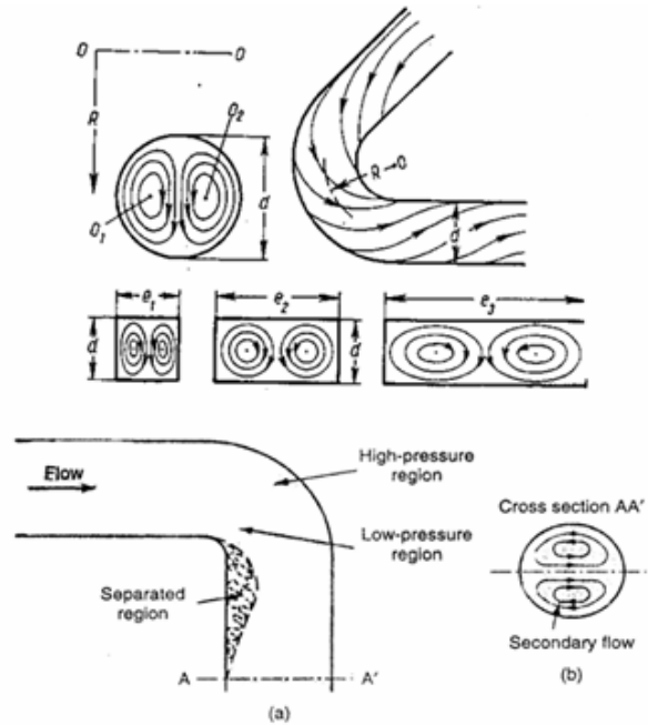
Gambar 7. Vortex Akibat Gaya Sentrifugal
