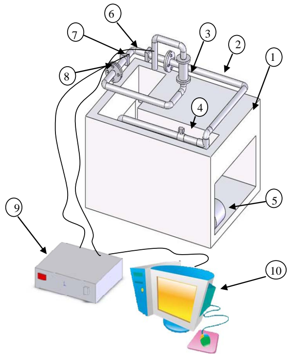
Gambar 3. Instalasi Peralatan Uji
