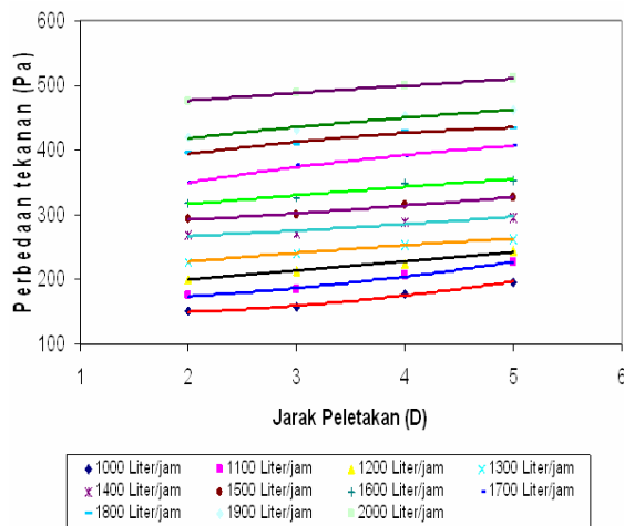
Gambar 8. Hubungan Antara Peletakan Tube Bundle dan Beda Tekanan
