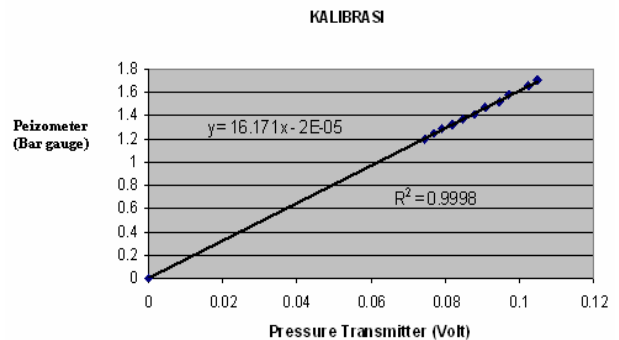
Gambar 4. Konversi Pressure Transmitter terhadap Piezometer
