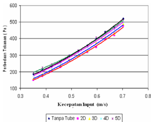
Gambar 6. Hubungan Antara Kecepatan Aliran Input dan Perbedaan Tekanan
