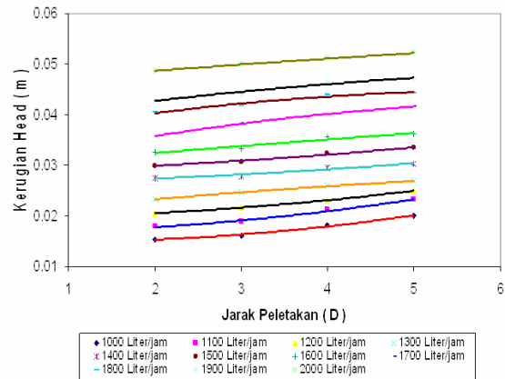
Gambar 9. Hubungan Antara Peletakan Tube Bundle dan Kerugian Head
