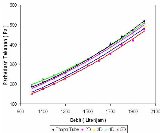
Gambar 5. Hubungan Antara Debit (Aliran) dan Perbedaan Tekanan
