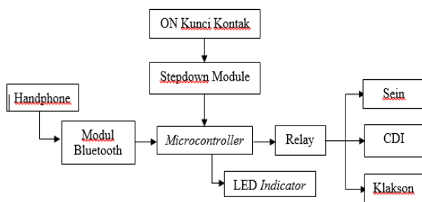
Gambar 3. Skema cara kerja sistem pengaman
