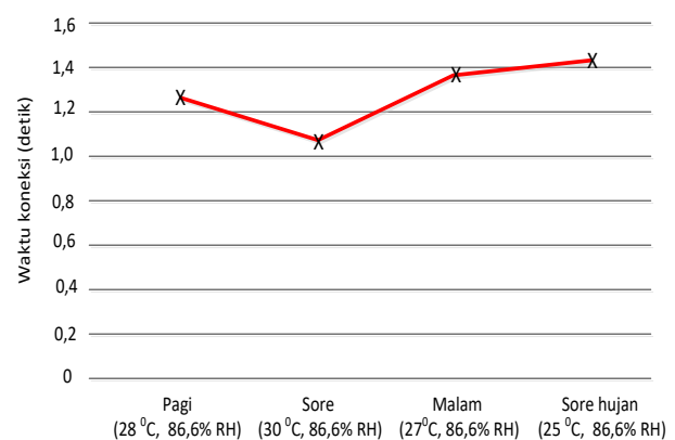
Gambar 5. Hasil uji keandalan sistem terhadap cuaca.
